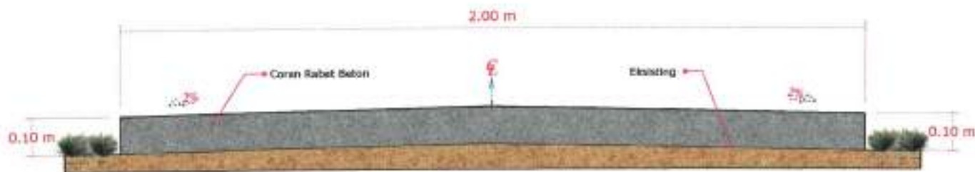
Jalan Rabet Beton Skala : 1:1000 s.d 1:300
